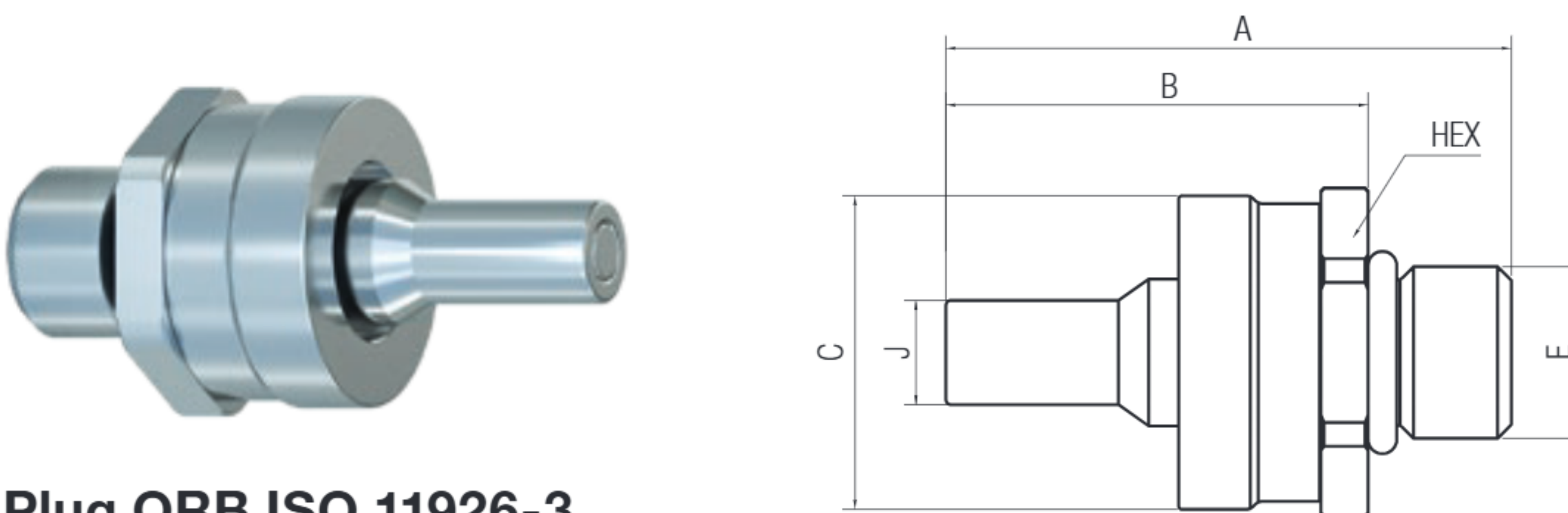
Plug ORB ISO 11926-3
