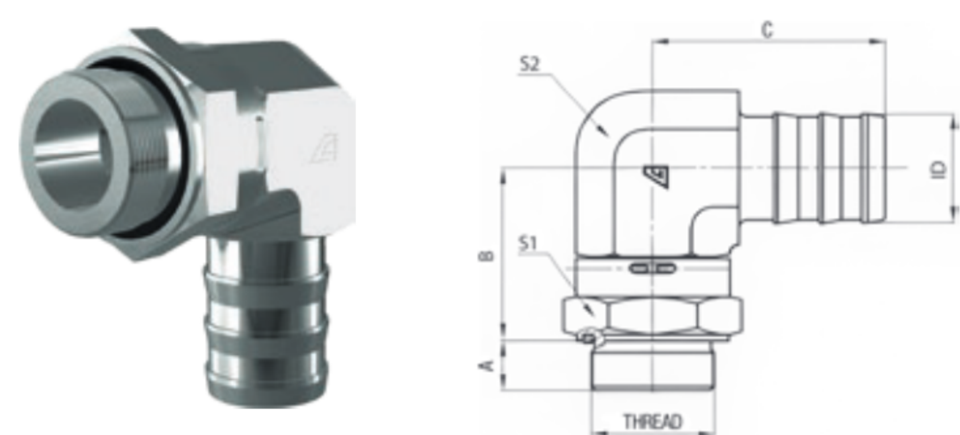
Port type ISO 1179-1
