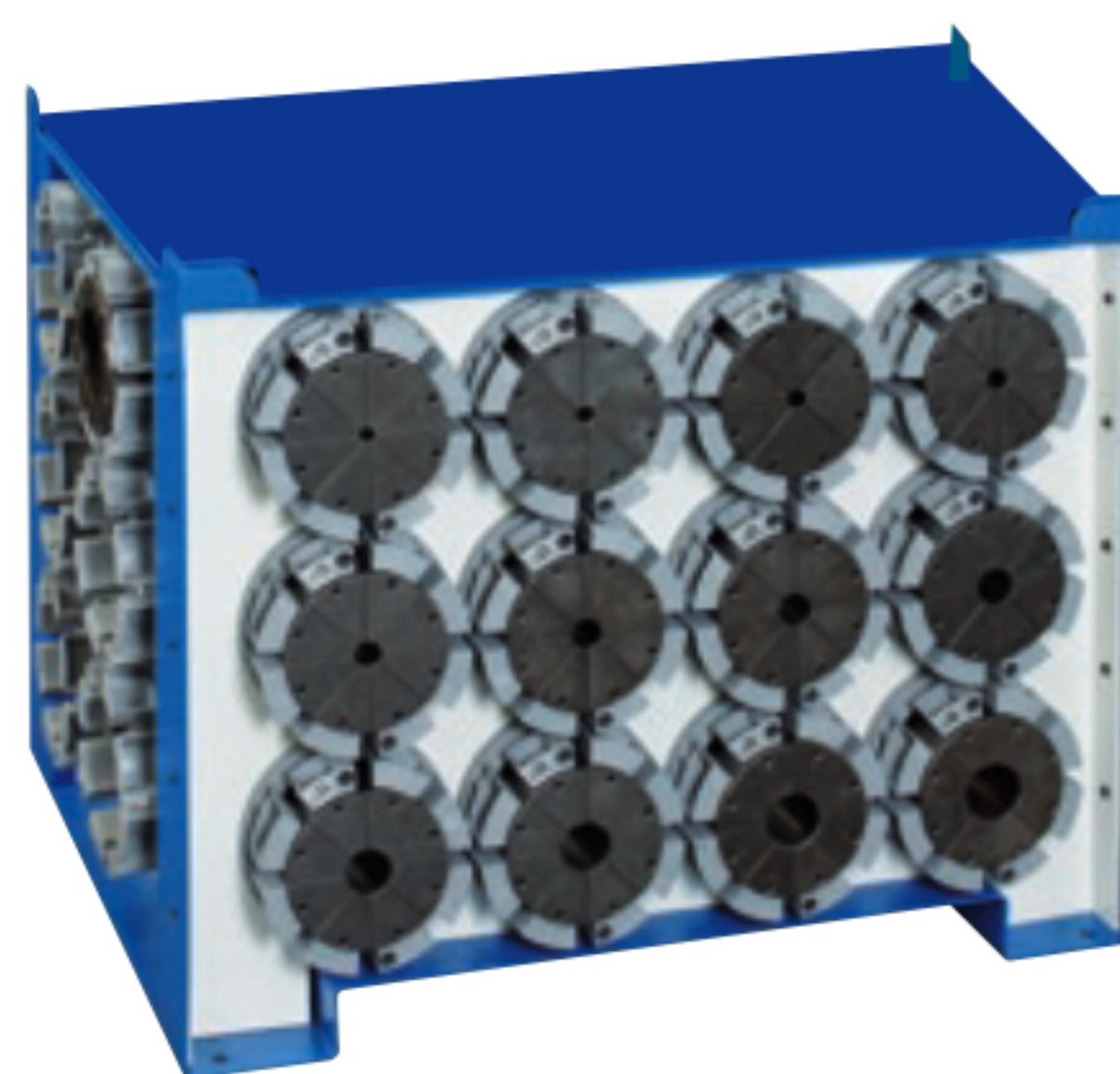
Die Base (18 PC.)
